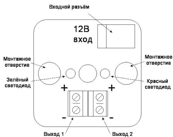
Внешний вид GC-0012U3 при снятой крышке
